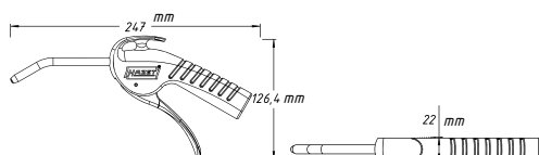
Standardní tryska
