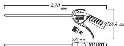
Dlouhá tryska
