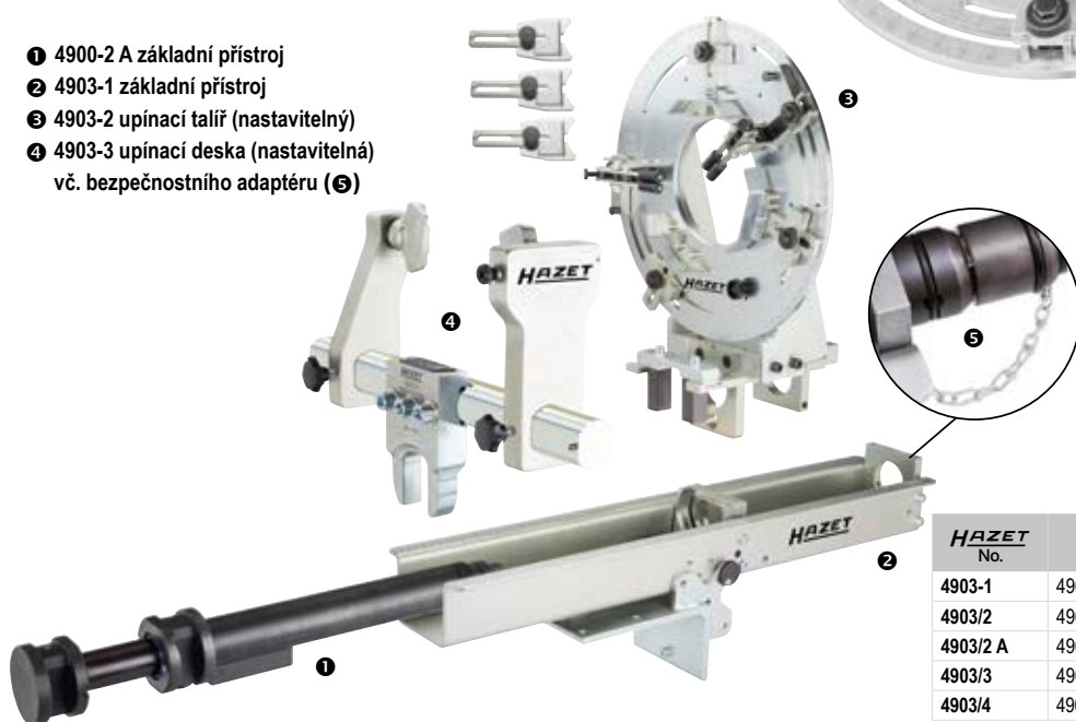
Stahovák pružin 4903/4
